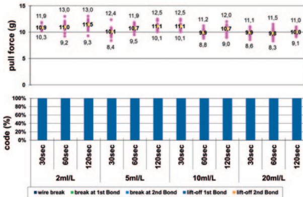
Abb. 4: Gute Bondbarkeit: der Golddraht-Bondtest zeigt deutlich höhere Abzugswerte als gefordert (lt. DSV 2611 min. Abzugswert 4 g)
