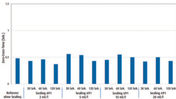
Abb. 5: Gute Lötbarkeit: Die Zero-Cross-Time im Lötwaagentest bleibt stabil unter einer Sekunde
