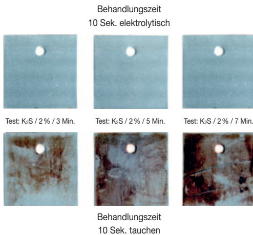
Abb. 1: Silberoberflächen mit Anlaufschutz: die elektrolytische Variante zeigt eine deutlich verbesserte K_2S -Beständigkeit
