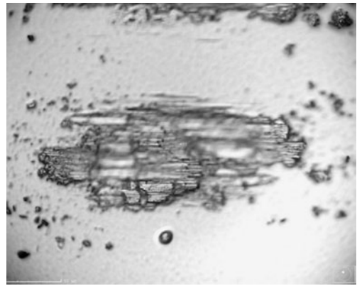
Silber-Reibspur Reibkoeffizient: 0,76
