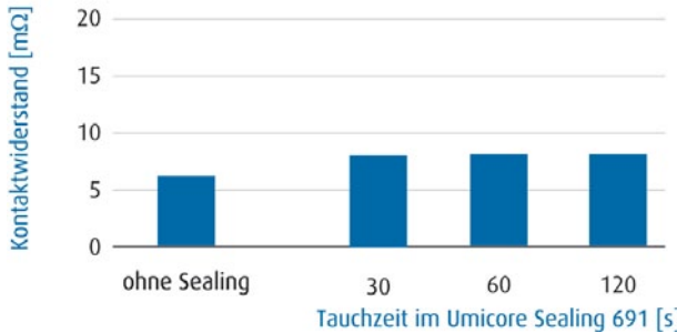
Abb. 3: Der Kontaktwiderstand bleibt stabil und zeigt keine Änderung durch die Anlaufschicht
